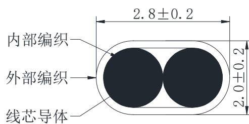
图 2 感应线截面示意图
